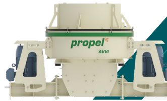
Vertical Shaft Impactor Seri AVVI Kapasitas : 40 TPH sampai 500 TPH Ukuran Pengumpanan (Maks.) : 32 sampai 66 mm
